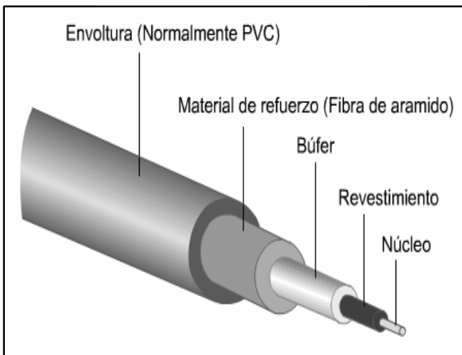
Imagen N° 4.1 Estructura del cable de fibra óptica
