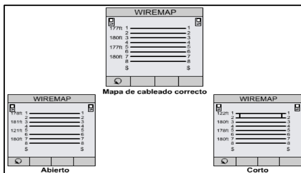
Imagen N° 11.1 Tipos de mapeo de cable UTP
