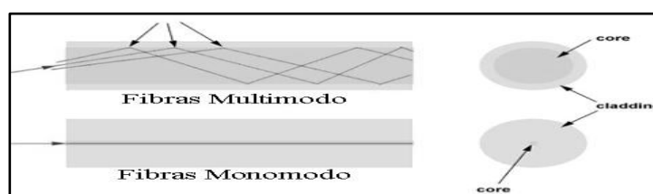
Imagen N° 3 Tipos de fibra óptica
