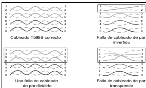
Imagen N° 11.2 Tipos de fallas cable UTP
