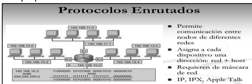
Imagen N° 35 Ejemplo de protocolo enrutado con su respectivo direccionamiento
