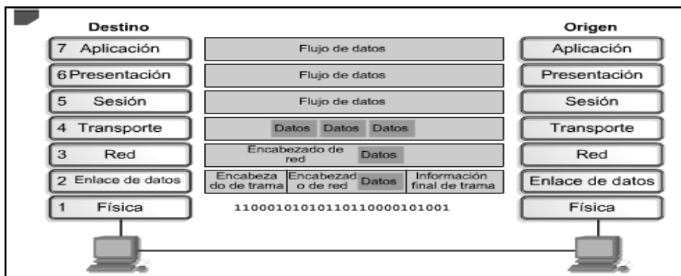
Imagen N° 14 Ejemplo del proceso de encapsulamiento
