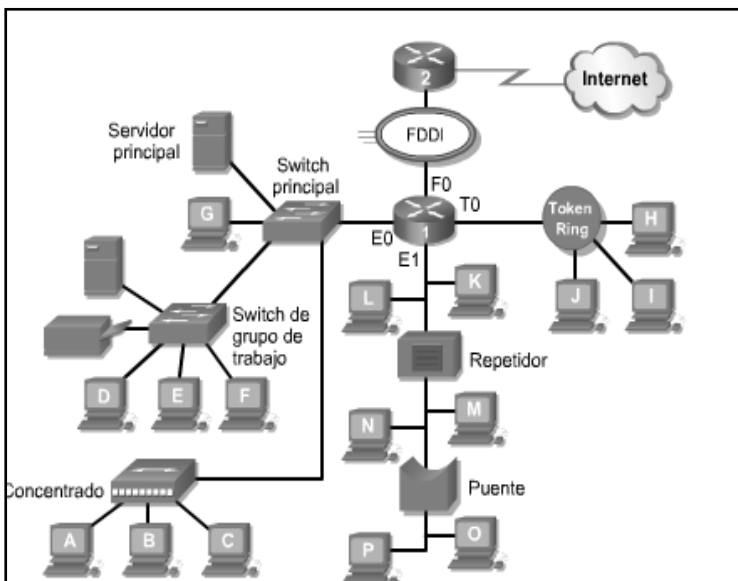
Imagen N° 14.2 Ejemplo de las diferentes redes, con diferentes topologías
