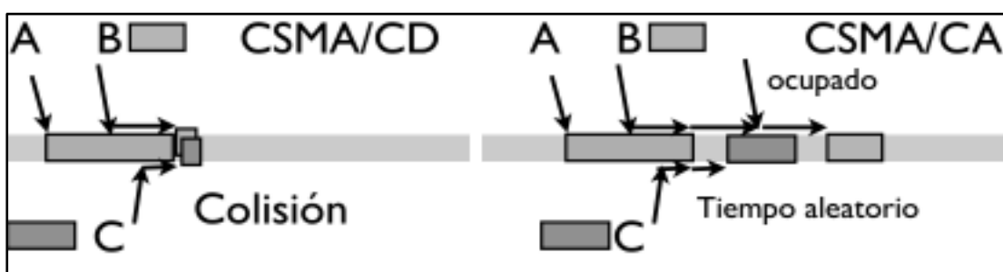
Imagen N° 14.3 Ejemplo de métodos de acceso al medio de Ethernet
