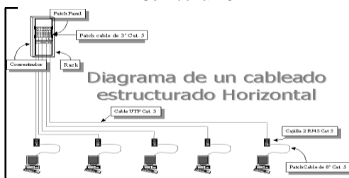
Imagen N° 6.1 Ejemplo de cableado horizontal Servidor a PC
