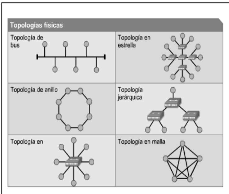
Imagen N° 14.1 Ejemplo de las diferentes topologías de red
