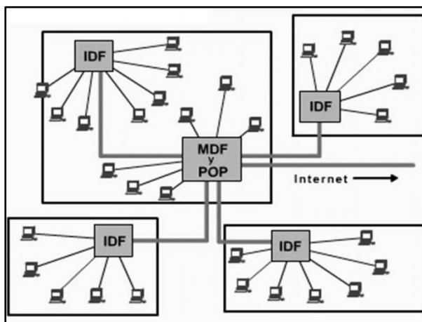
Imagen N° 8.1 Ejemplo de cableados verticales Y horizontales mediante MDF E IDF
