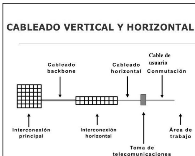
Imagen N° 7.2 Ejemplo de conexiones entre cableado vertical y cableado horizontal
