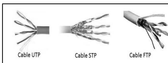
Imagen N° 2.1 Tipos de cable UTP
