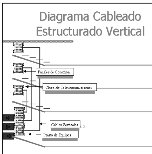
Imagen N° 7.1 Ejemplo de cableado vertical Rack primario a rack secundarios
