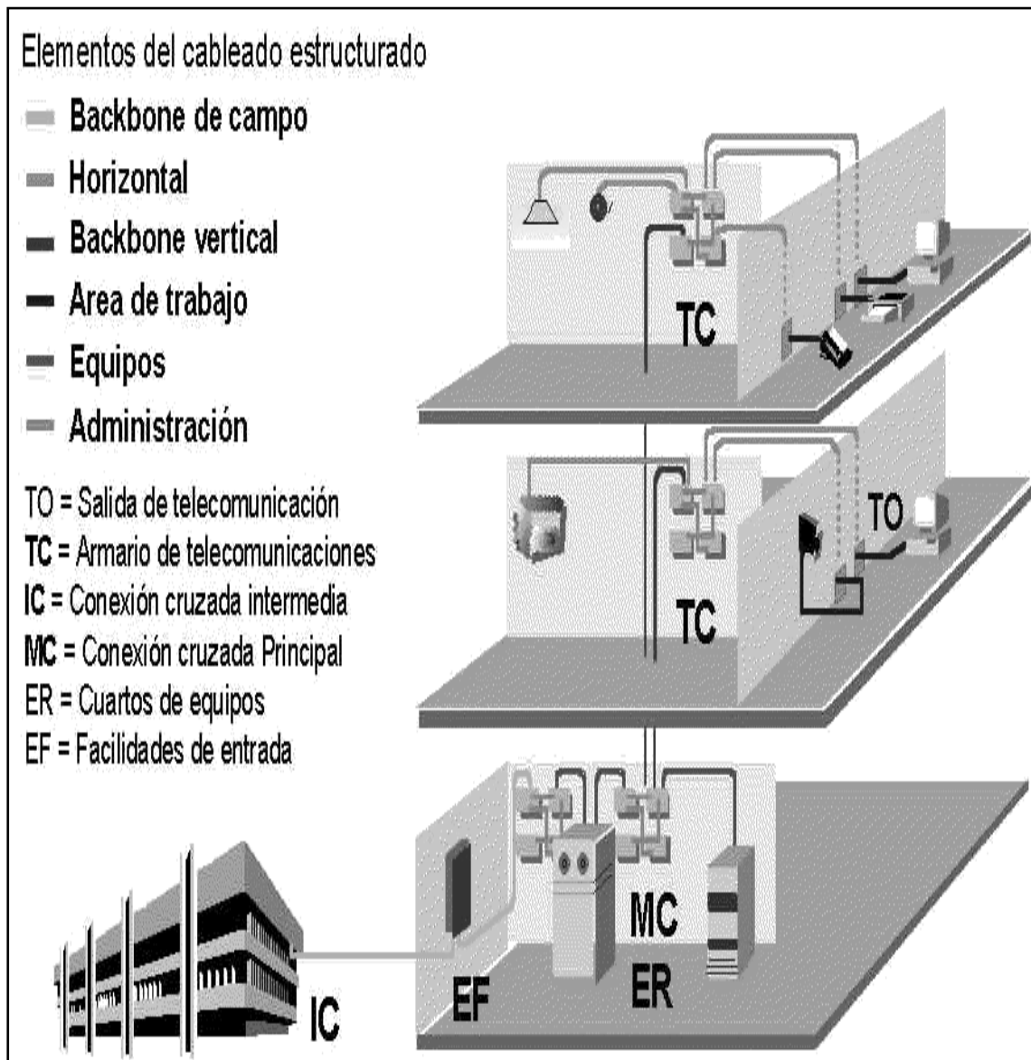
Imagen N° 5 Estructura funcional de un cableado estructurado
