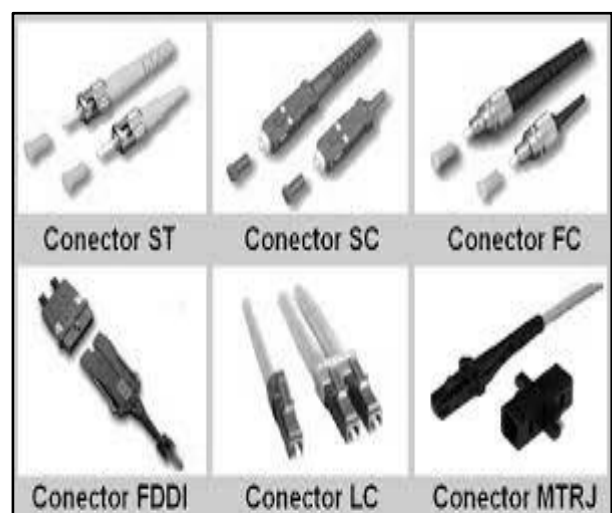
Imagen N° 4.2 Tipos de fibra óptica
