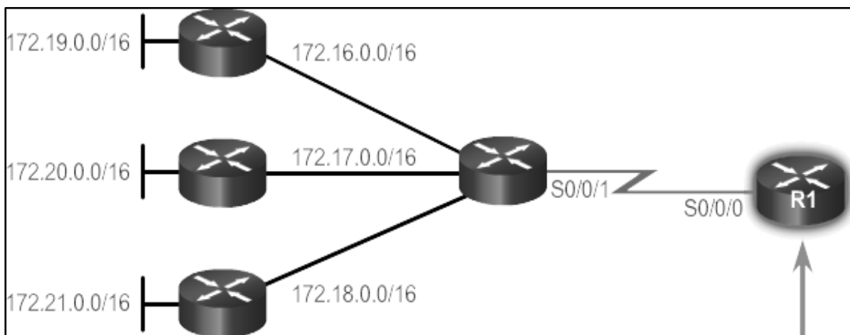
Imagen N° 19 Ejemplo de CIDR en una dirección IPV 4 clase c
