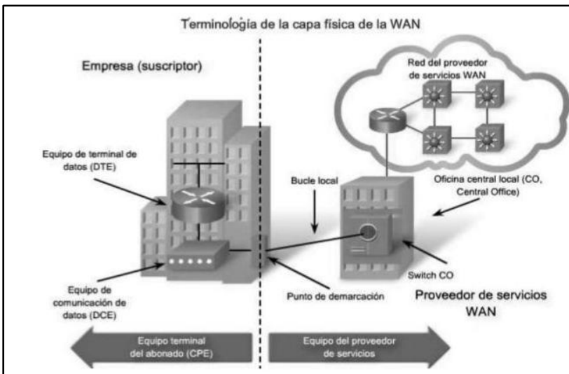
Imagen N° 10.1 Ejemplo de límite de la responsabilidad del servicio entre la empresa (ISP) y el usuario
