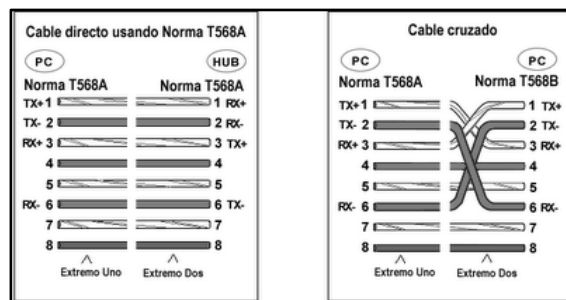
Imagen N° 11.1 Muestra una conexión directa y cruzada de un cable UTP
