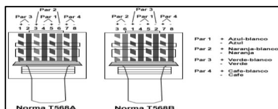
Imagen N° 2.2 Estructura de cable UTP
