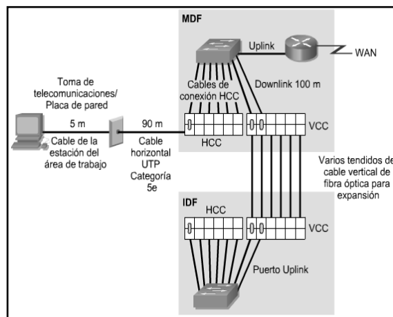
Imagen N° 8.2 Ejemplo de una estructura topológica, mediante cableado horizontal y vertical
