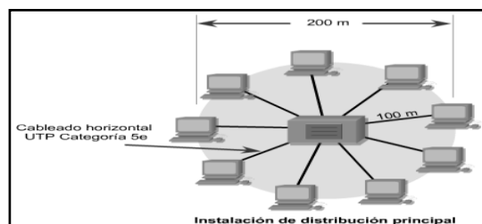
Imagen N° 6.2 Ejemplo de cableado horizontal Switches a PC
