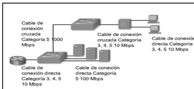
Imagen N° 10.2 Ejemplo de directas y cruzadas con diferentes dispositivos de red
